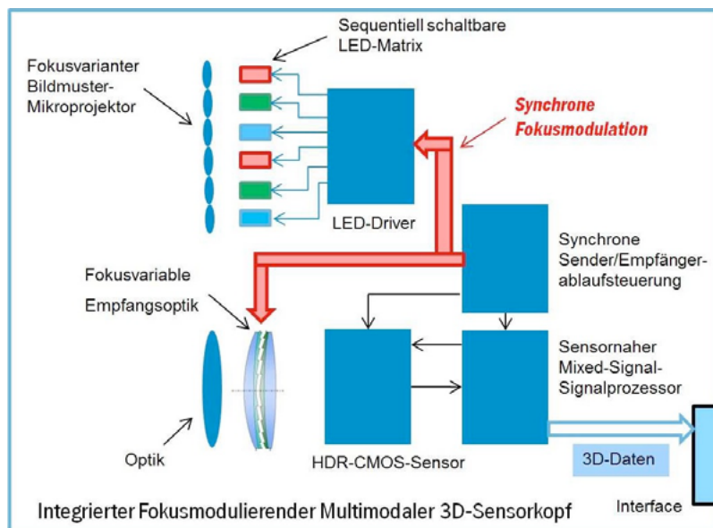
Bild 2: Prinzipskizze des 3D-Sensorkopfs. (Quelle: Sick AG)
